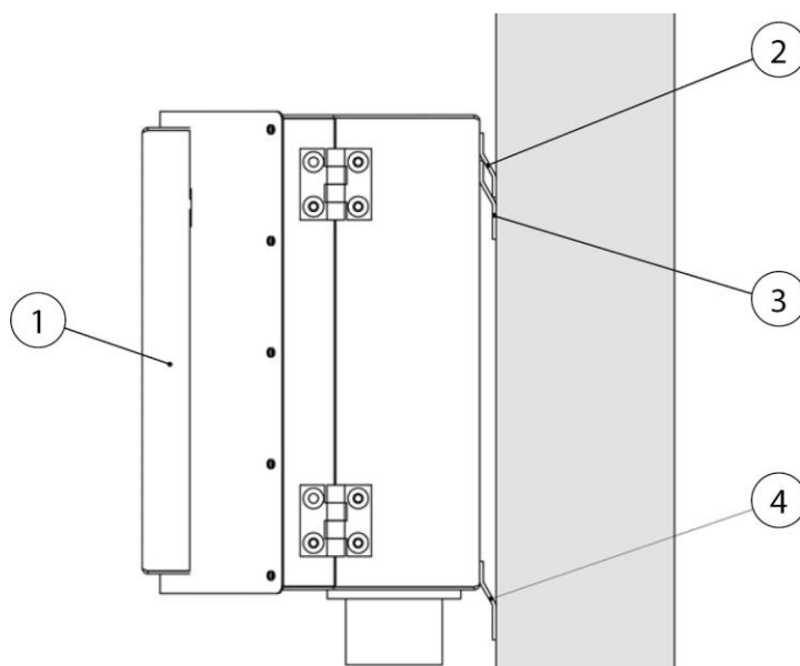
Bild 8: Montera kontrollboxen
