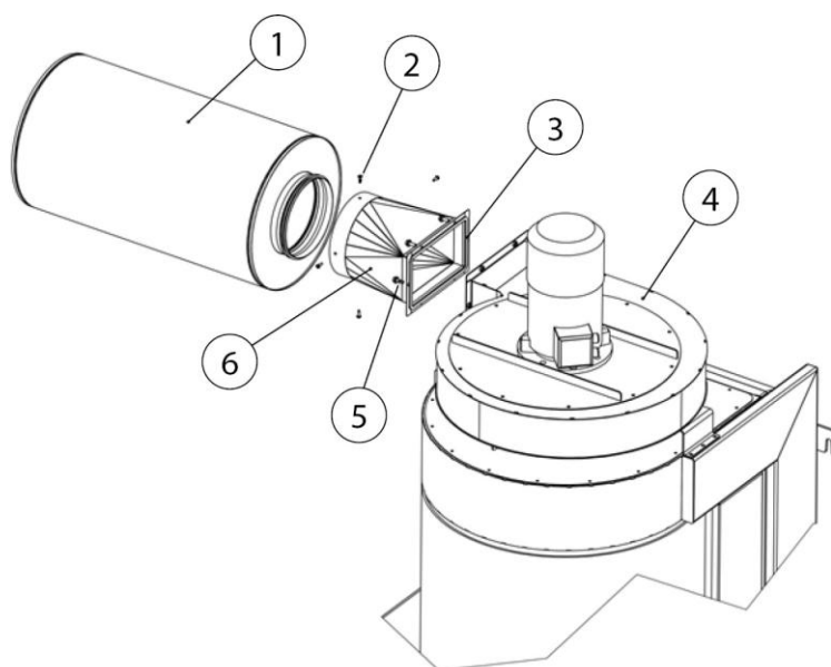
Bild 6: Montera ljuddämpare
