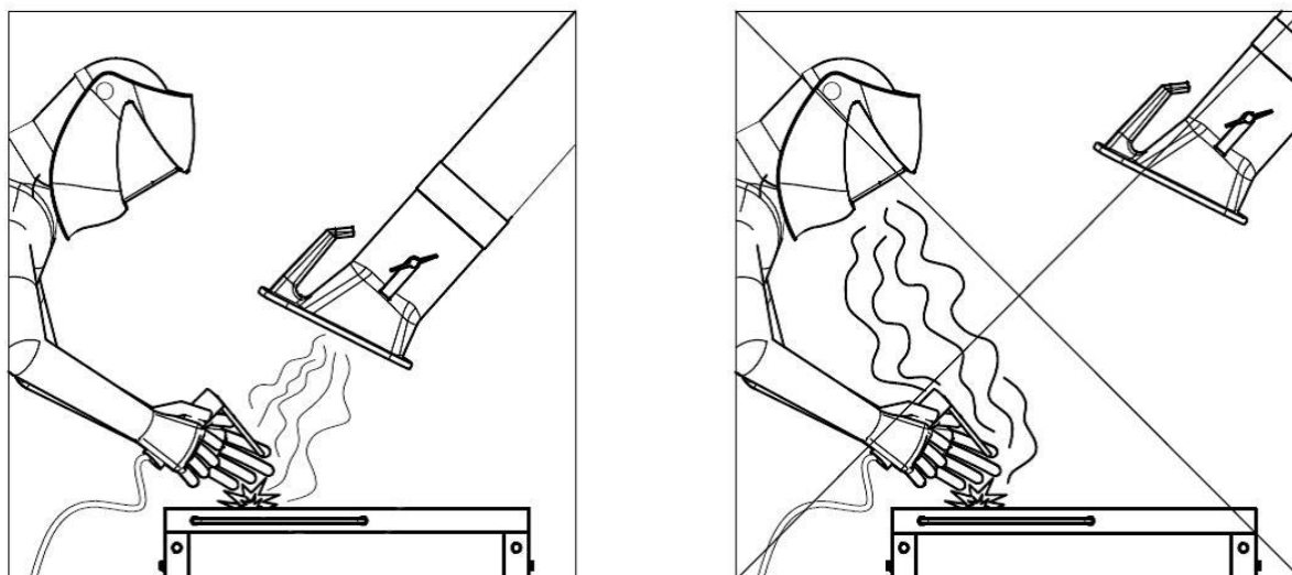
Bild 11: Positionering av sugkåpan
