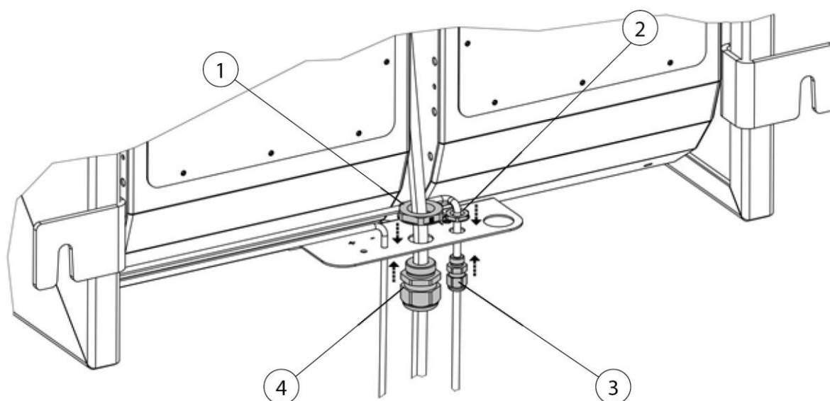
Bild 5: Montera kabelförskruvningar
