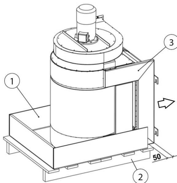
Bild 4: Montera produkten
